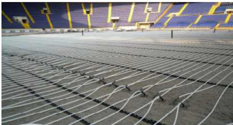
Rys. 10 Montaż podziemnego systemu grzewczego.
